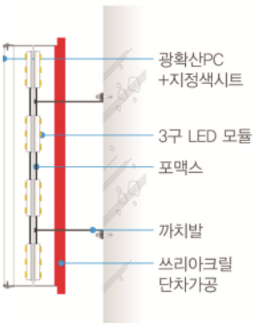
- 전후광채널 단면도
