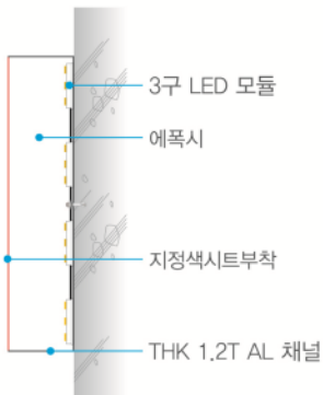
- 에폭시채널 단면도
