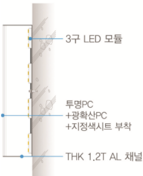
- 알루미늄 일체형채널 단면도
